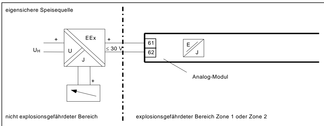
Bild 13 Analog-Modul Ex
