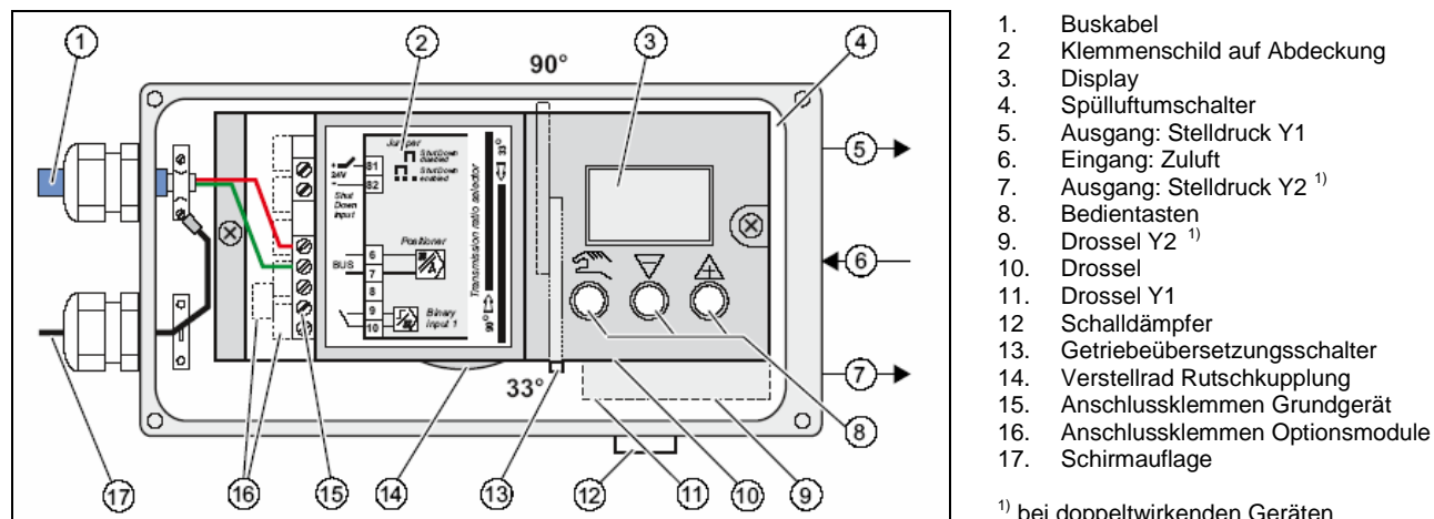
Bild 1 Aufbau
