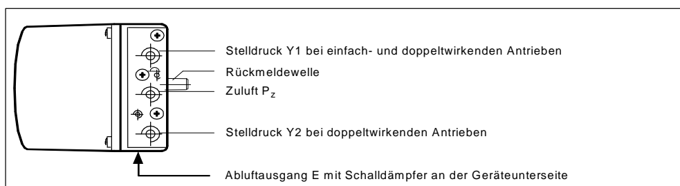
Bild 21 Pneumatischer Anschluss
