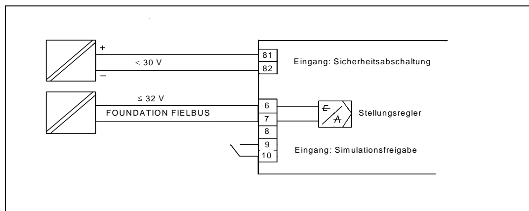
Bild 8 Elektrischer Anschluss Grundgerät nicht ex
