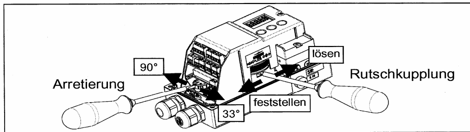
Bild 3 Arretierung von Rutschkupplung und Getriebeübersetzungsschalter
