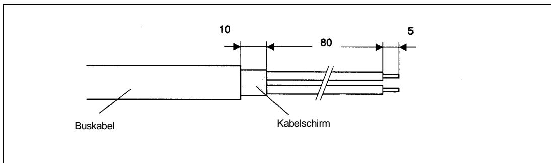
Bild 10 Vorbereitung des Buskabel
