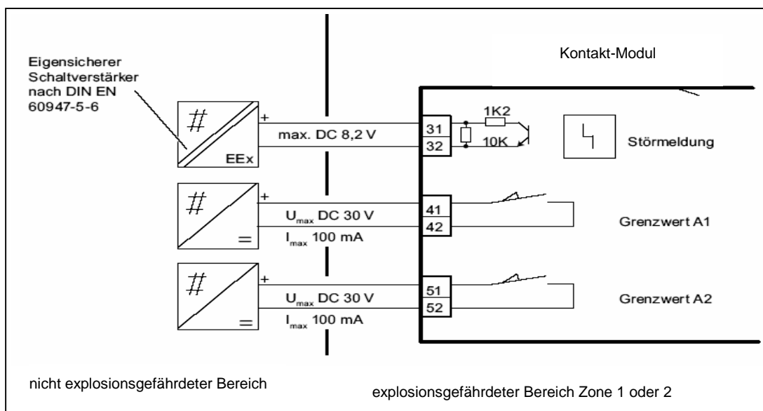
Bild 19 Kontakt-Modul ex
