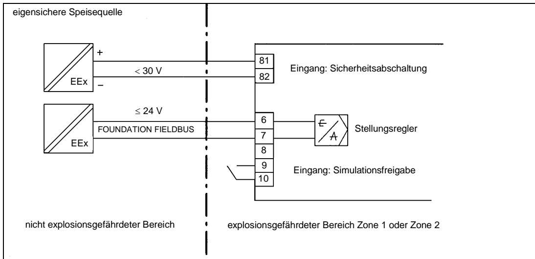
Bild 9 Elektrischer Anschluss Grundgerät ex
