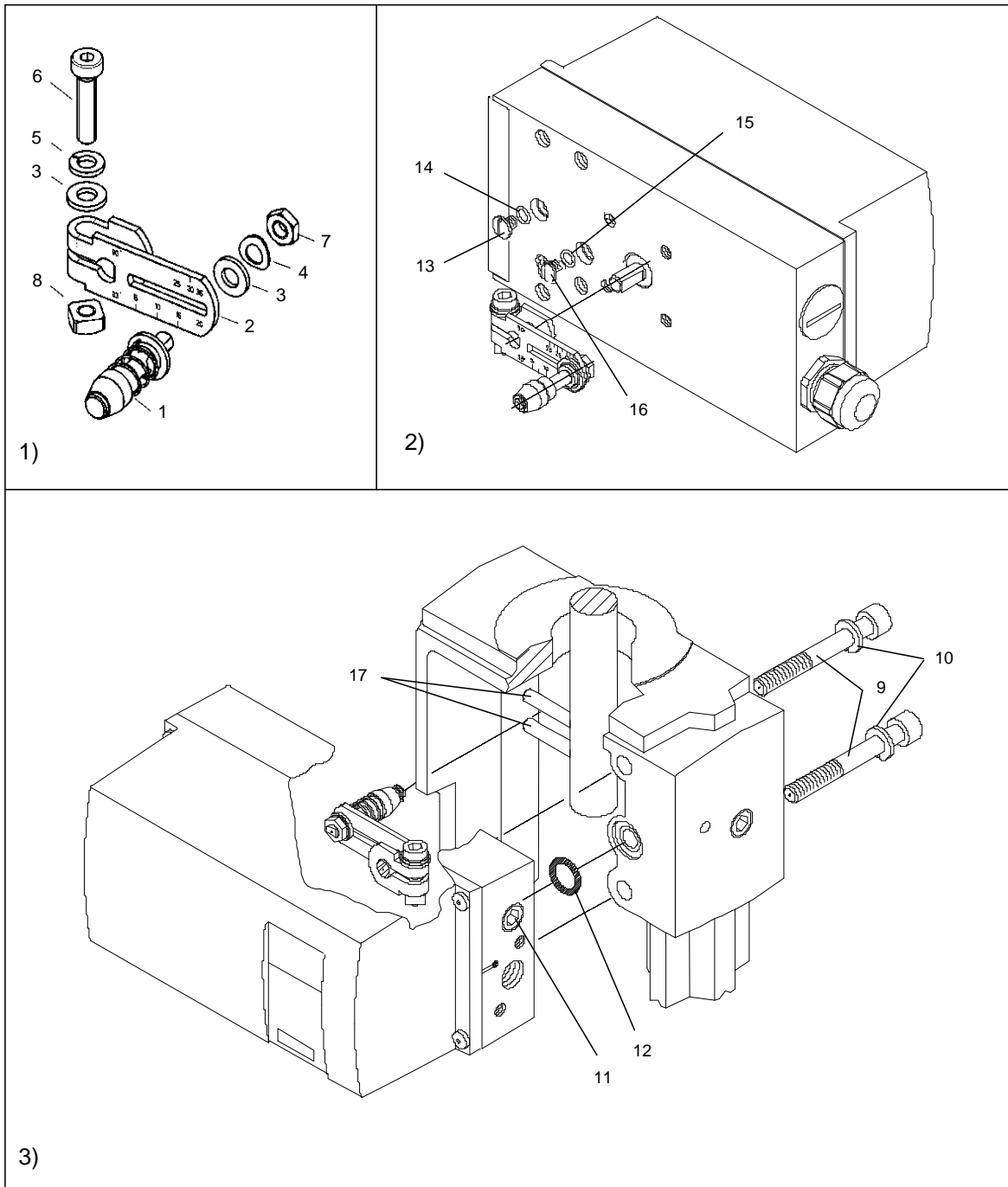
Bild 4 Montageablauf integrierter Anbau
