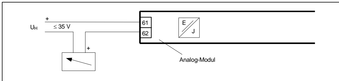
Bild 12 Analog-Modul nicht Ex
