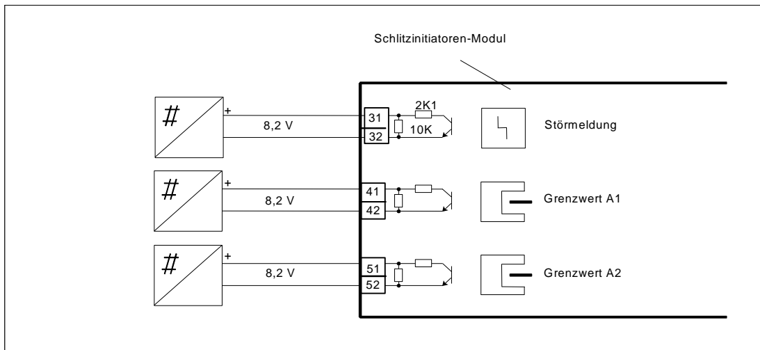
Bild 16 Schlitzinitiatoren-Modul nicht Ex
