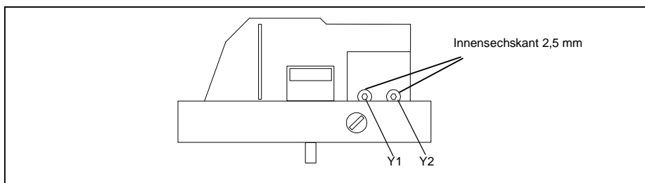
Bild 23 Drosseln
