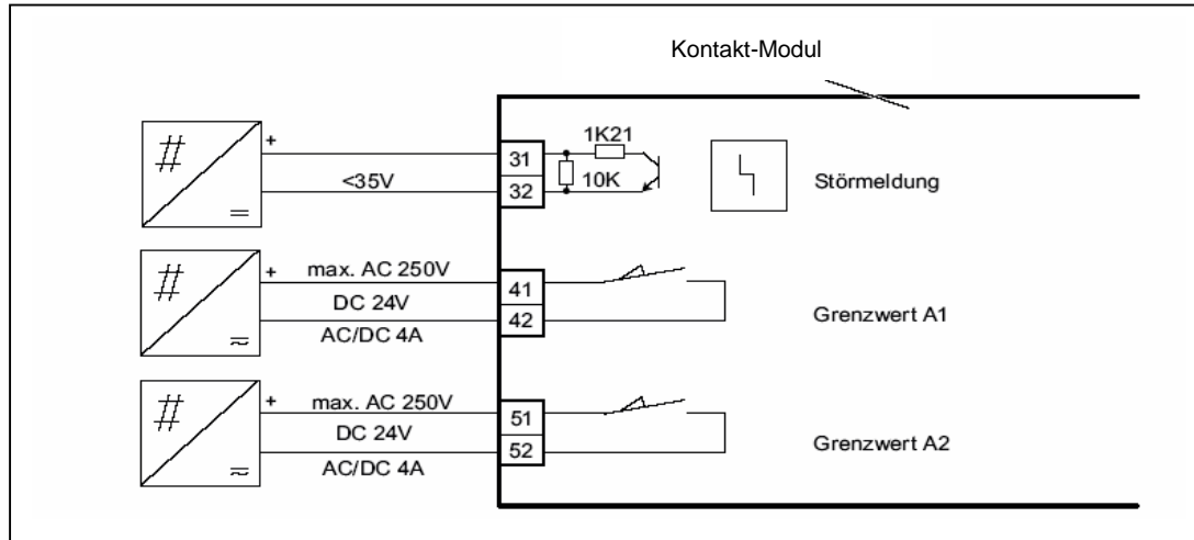
Bild 18 Kontakt-Modul nicht ex
