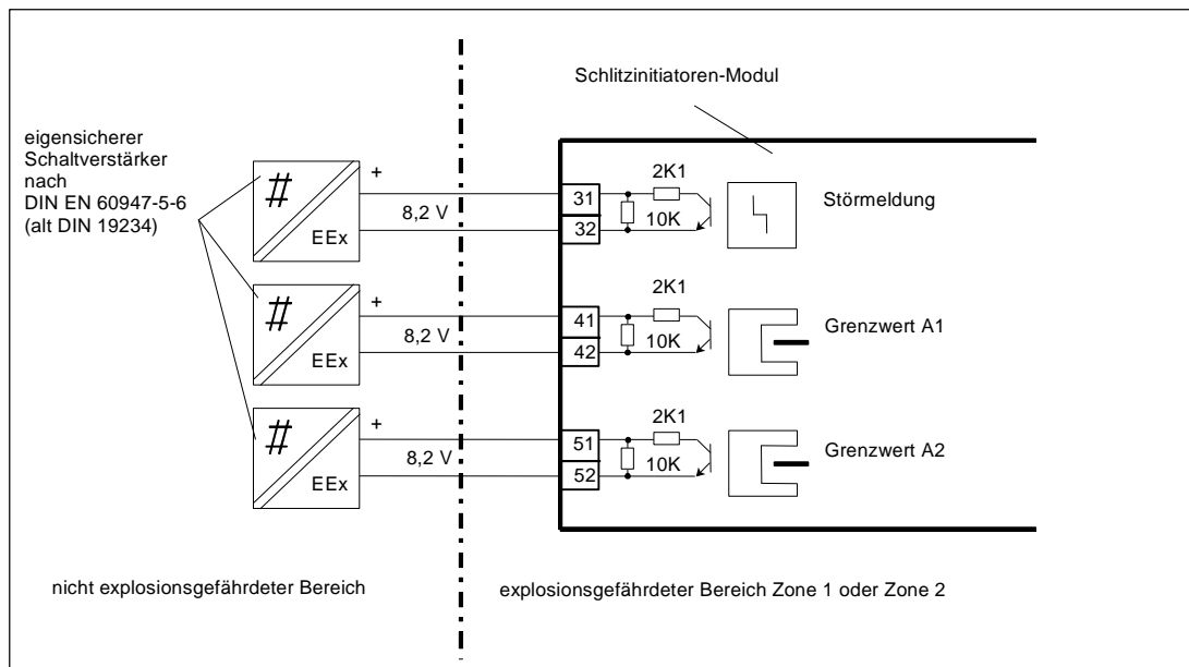
Bild 17 Schlitzinitiatoren-Modul Ex
